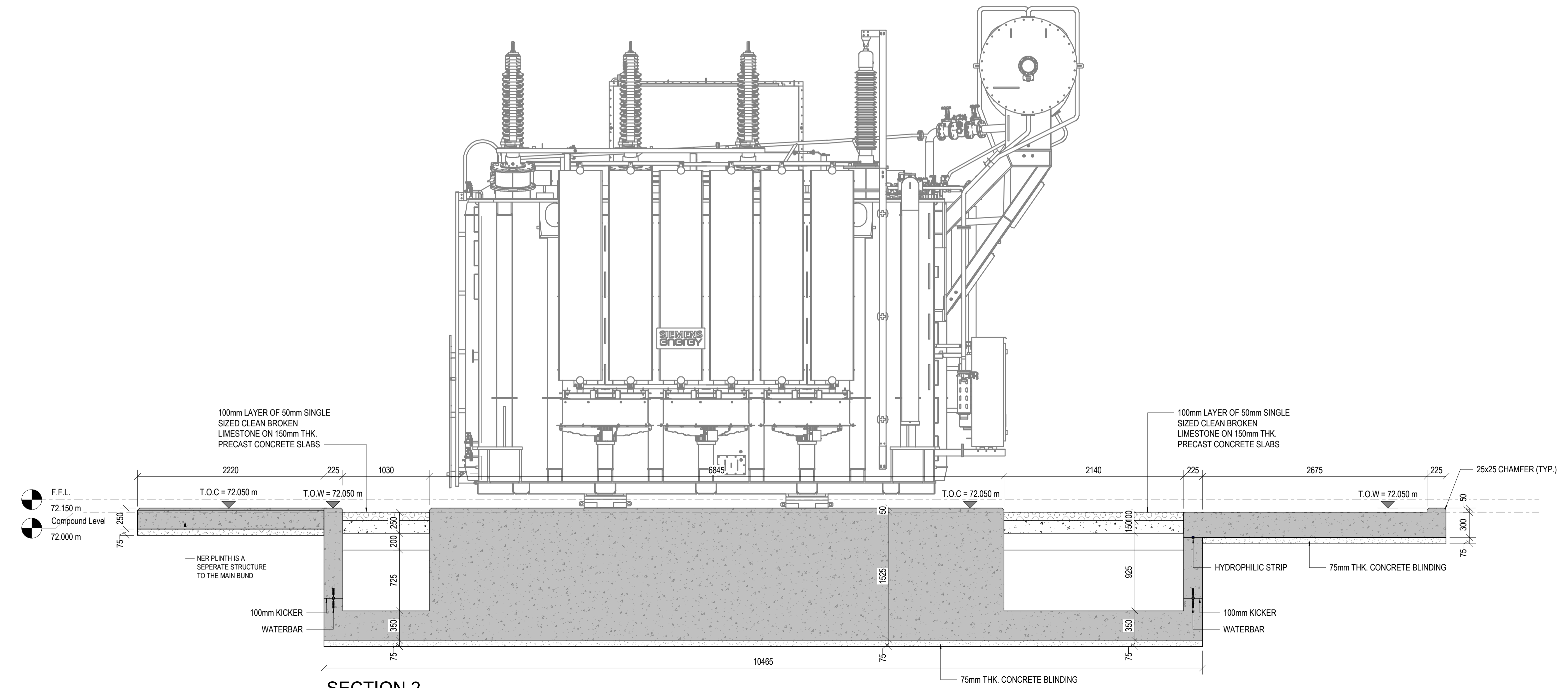
SECTION 2 SCALE 1 : 30
