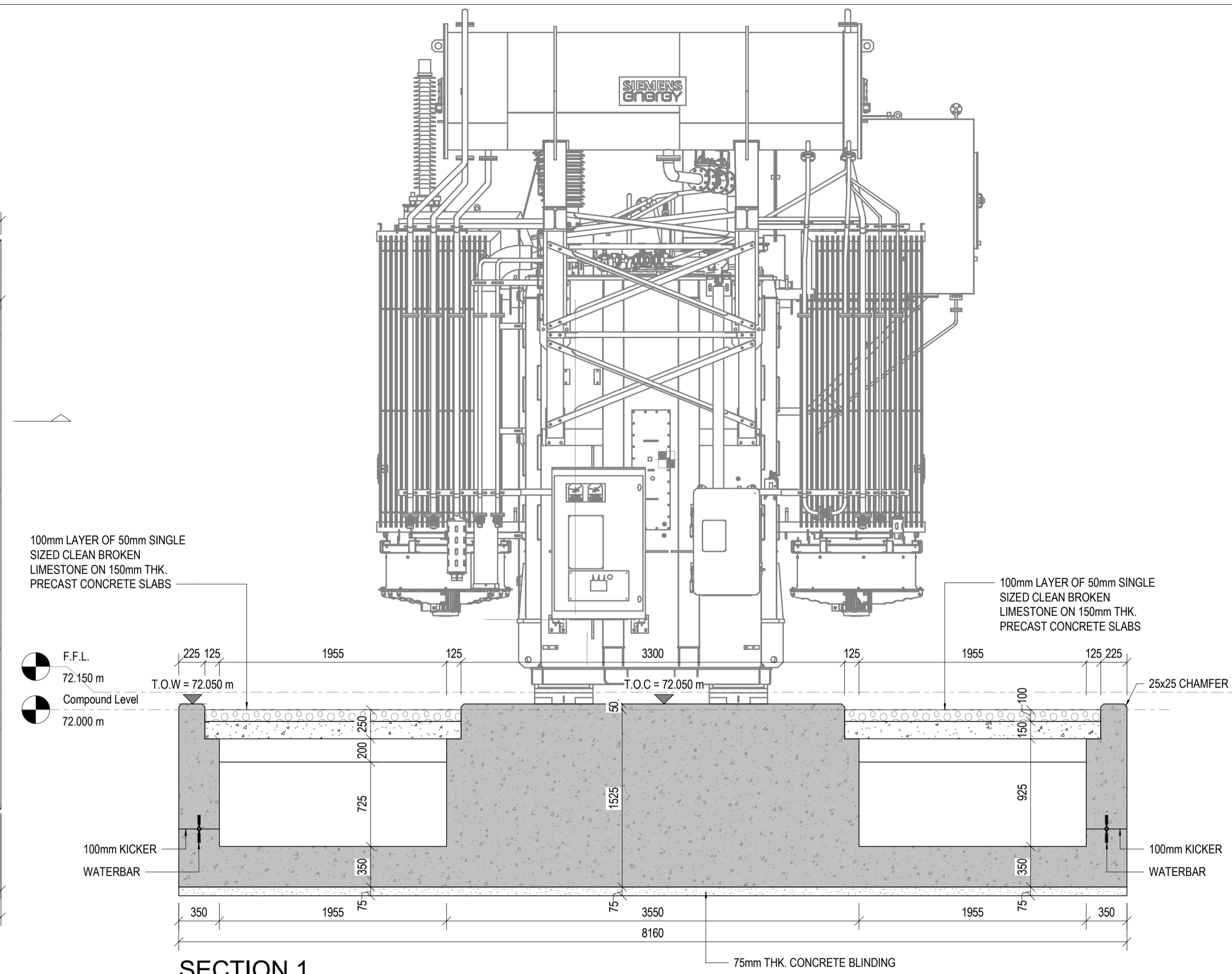
SECTION 1 SCALE 1 : 30
